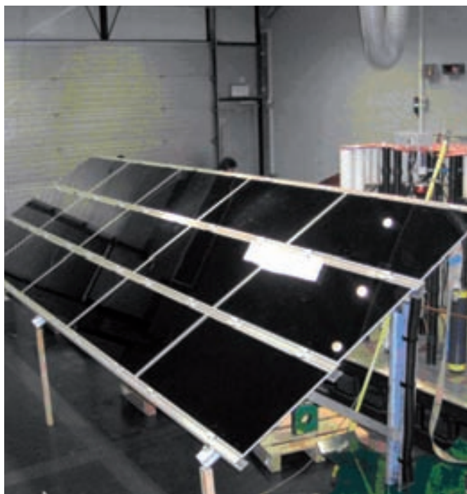
Fig. 6 : Laboratoire DEHN : Montage expérimental pour tester des surtensions induites dans un champ de modules provoquées par le champ magnétique généré par un courant de foudre à proximité
