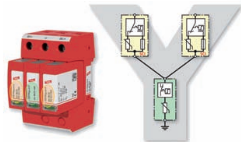
Fig. 10 : SPD avec "montage en étoile résistant aux défauts"
