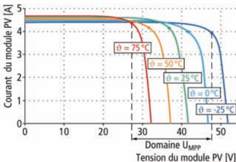
Fig. 8 : Caractéristique courant-tension d'un module PV pour différentes températures des cellules
