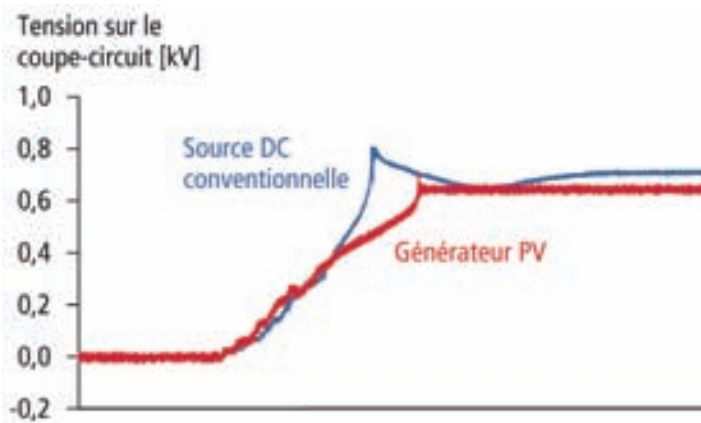
Fig. 12 : Essai comparatif de la coupure du courant continu d'une source de courant continu conventionnelle et d'un générateur PV réel
