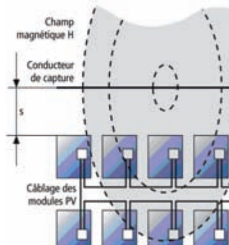
Fig. 4 : Surtensions induites dans un champ de modules provoquées par le champ magnétique généré par un courant de foudre à proximité
