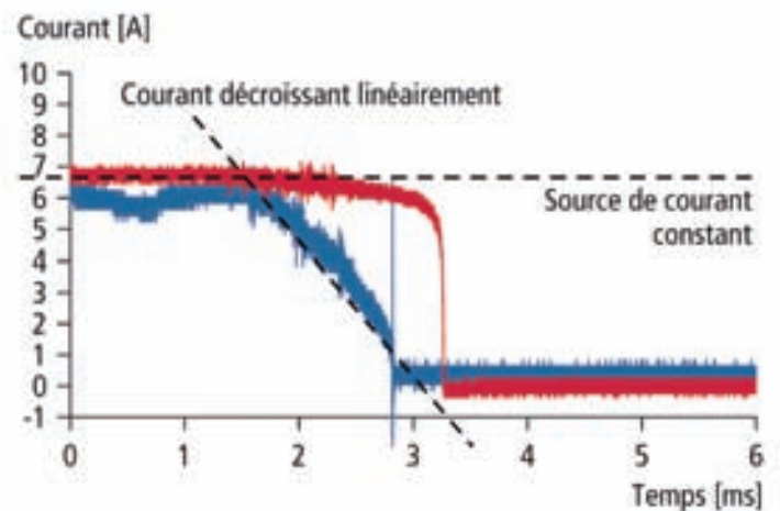
Fig. 12 : Essai comparatif de la coupure du courant continu d'une source de courant continu conventionnelle et d'un générateur PV réel
